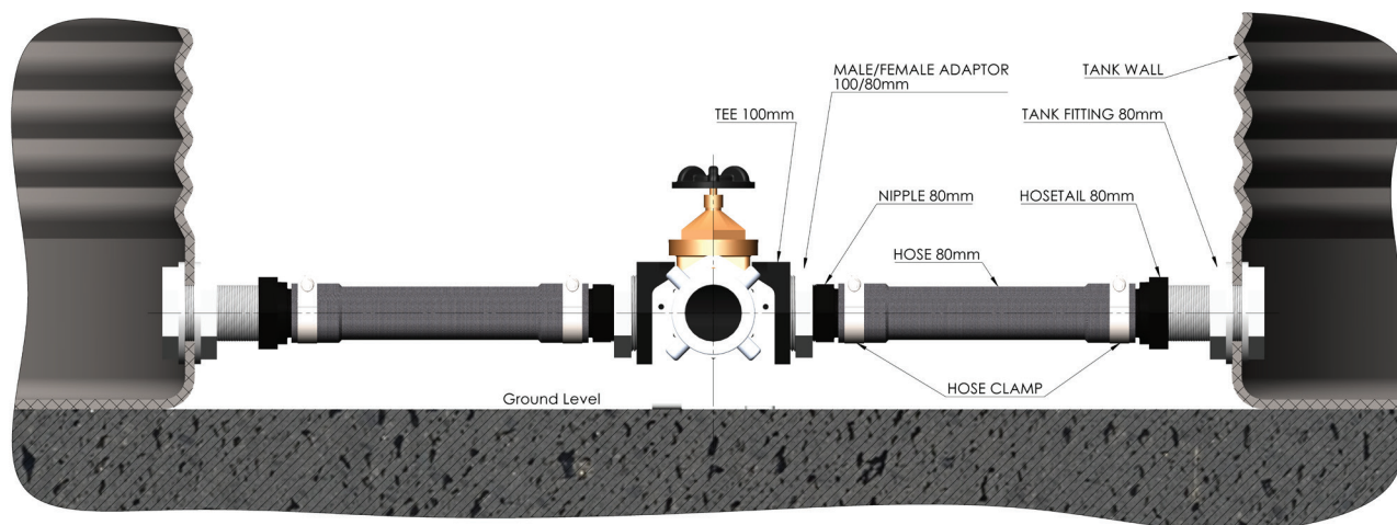
SECTION B-B SCALE 1 : 5
