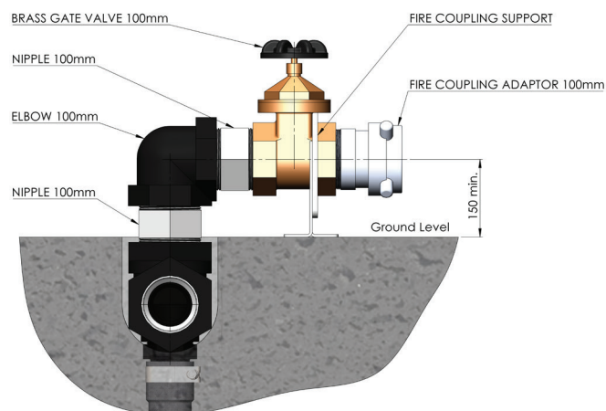
SECTION A-A SCALE 1 : 5
